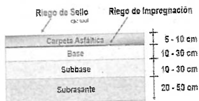
Imagen N°01: Corte Transversal de la Estructura del Pavimento
